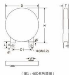
(图1: 40D系列简图)
